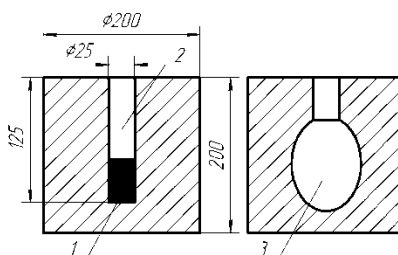
1 – заряд ВВ; 2 – исходная полость; 3 – полость после взрыва
